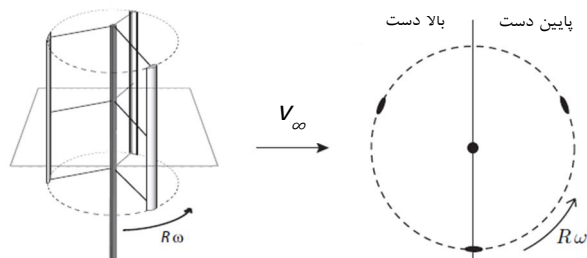
الف- تصویر دو بعدی مقطع توربین ب- شماتیک سه بعدی توربین
