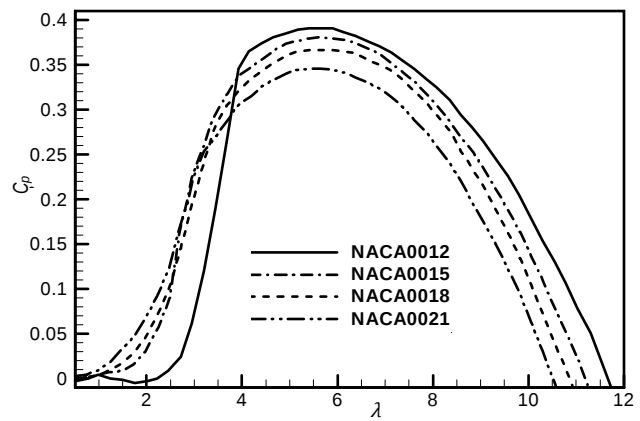
شکل 8 تغییر ضخامت پره بر منحنی ضریب توان
