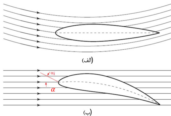
شکل 11 جریان اطراف ایرفویل الف-حالت واقعی ب- حالت معادل مقابل باد مستقیم
