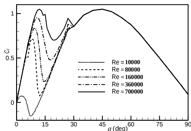
شکل 9 تغییرات ضریب برآ برحسب زاویه در چند عدد رینولدز مختلف [11]
