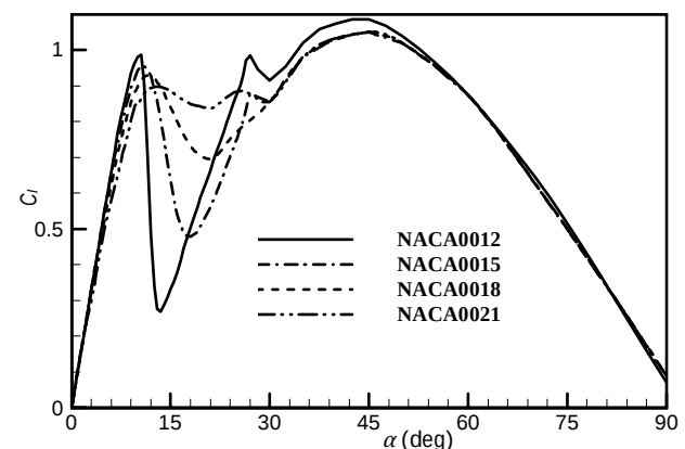
شکل 10 تغییرات ضریب برآ با زاویه حمله برای چند پره مختلف [11]
