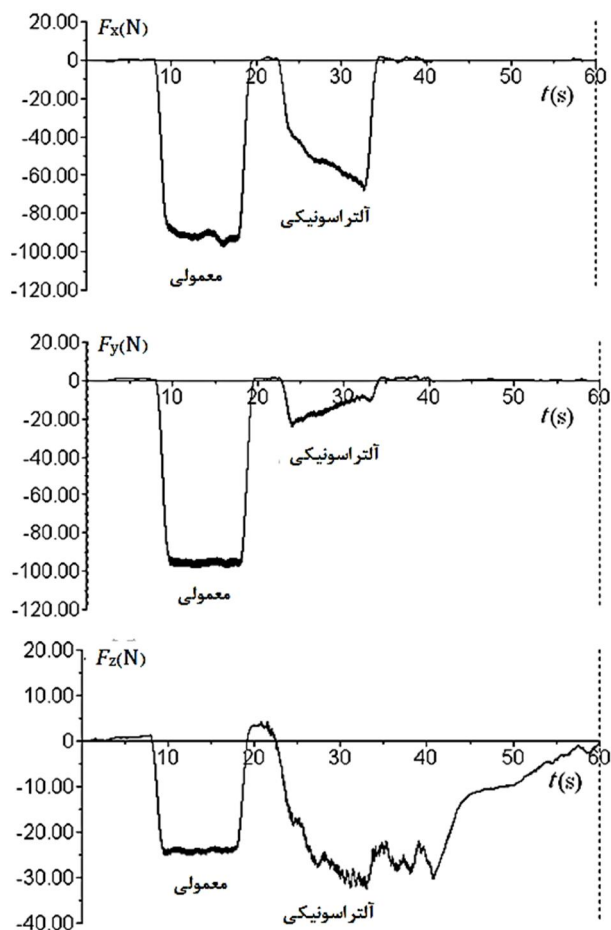
شکل 3 نمونه ای از نیروهای اندازه گیری شده توسط دینامومتر با شرایط rpm a=24 \mu m و a_r=1/5 mm ، f_z=0/15 mm/tooth ، N=400
