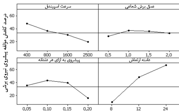
شکل 4 تأثیر سرعت اسپیندل، پیشروی به ازای هر دندانه، عمق برش شعاعی و دامنه ارتعاش بر درصد کاهش مؤلفه پیشروی نیروی برشی در فرزکاری آلتراسونیک نسبت به فرزکاری معمولی
