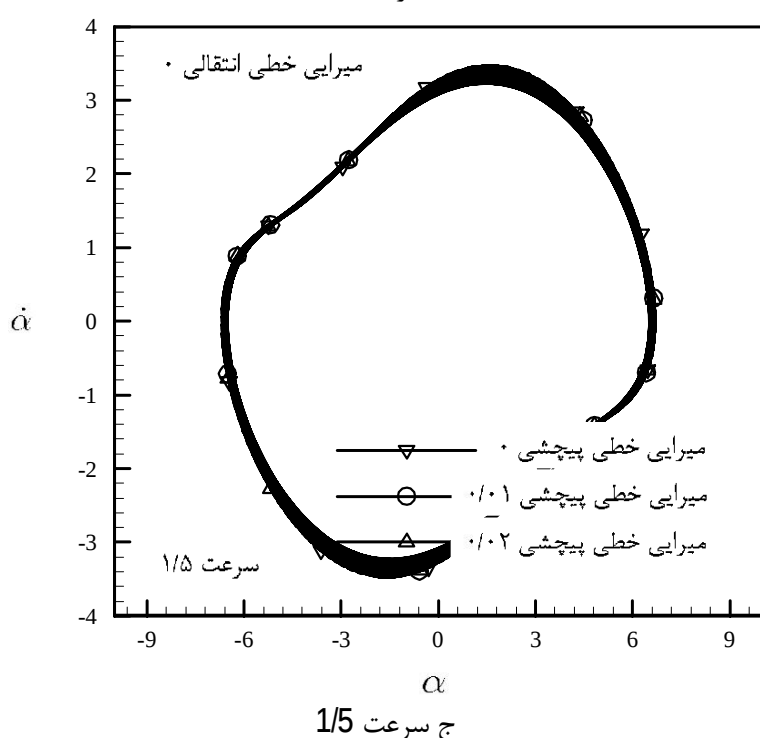
شکل 11 نمودار فازی بالک غیرخطی براساس تغییر میرایی خطی پیچشی (\zeta_\alpha=0, 0.01, 0.02) ، برای میرایی انتقالی (\zeta_h=0) و سفتی پیچشی و انتقالی (\hat{\eta}_h=5, \hat{\eta}_\alpha=5) و اثر لقی (\alpha_s=1^\circ, \zeta_s=0.05)
