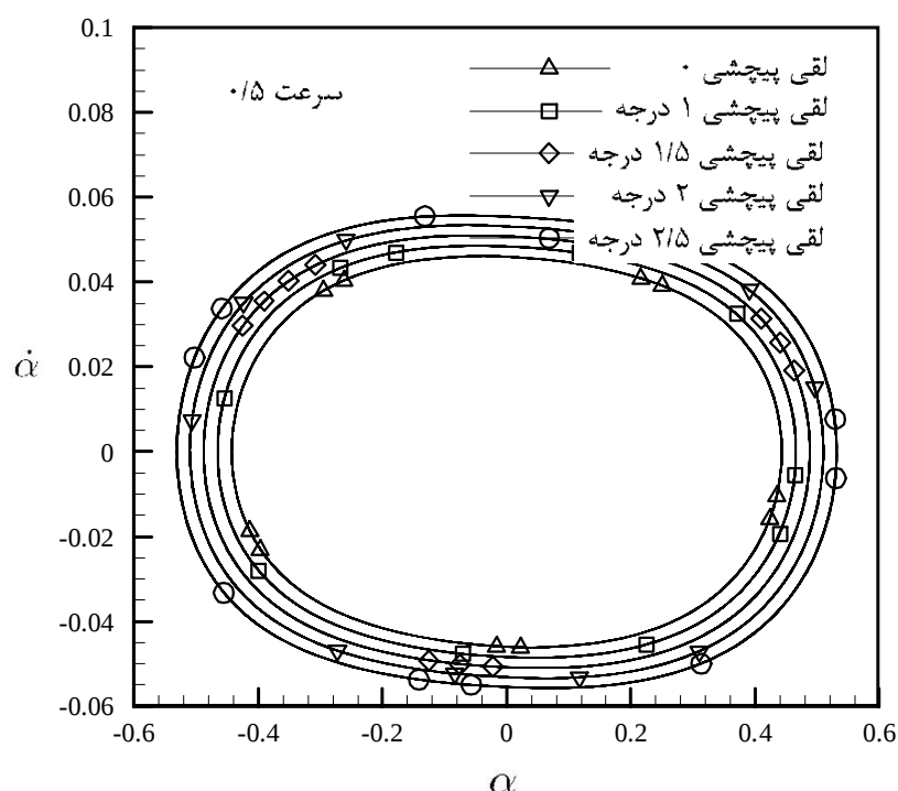
شکل 13 نمودار فازی برای سرعت 0/5، سفتی پیچشی و انتقالی ( \hat{\eta}_h = 10, \hat{\eta}_\alpha = 10 ) و اثر لقی ( \xi_s = 0, \alpha_s = 0, 1^\circ, 1.5^\circ, 2^\circ, 2.5^\circ )
