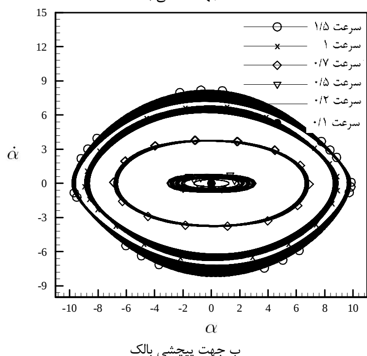
شکل 6 نمودار فازی بالک الاستیک با سفتی غیرخطی انتقالی ( \hat{\eta}_h=10, \hat{\eta}_\alpha=0 ) بدون اثر لقی ( \xi_s=\alpha_s=0 ) و میرایی ( \zeta_h=\zeta_\alpha=0 )
