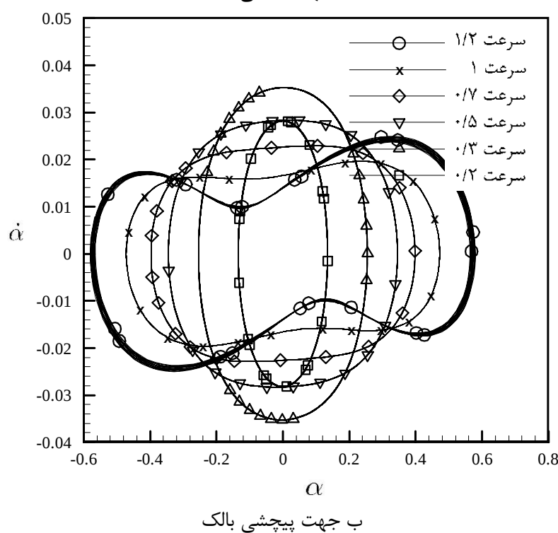
شکل 7 نمودار فازی بالک الاستیک با سفتی غیرخطی پیچشی ( \hat{\eta}_h=0, \hat{\eta}_\alpha=10 ) بدون اثر لقی ( \xi_s=\alpha_s=0 ) و میرایی ( \zeta_h=\zeta_\alpha=0 )
