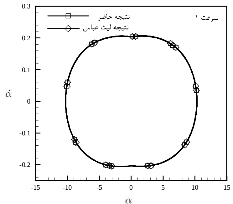
شکل 4 مقایسه نمودار فازی حرکت پیچشی با ضخامت ( \hat{\tau}=0.095 )، اثر لقی ( \hat{\eta}_h=0, \hat{\eta}_\alpha=10 ) و سفتی پیچشی ( \xi_s=0, \alpha_s=0.5^\circ )
