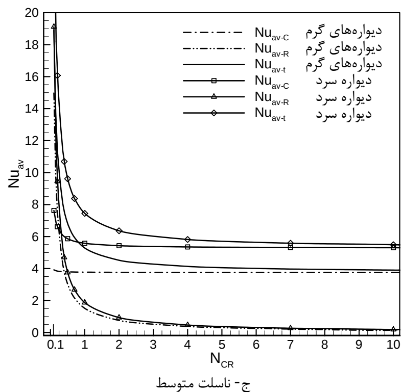
شکل 14 تغییرات عدد ناسلت برحسب عدد پلانک
