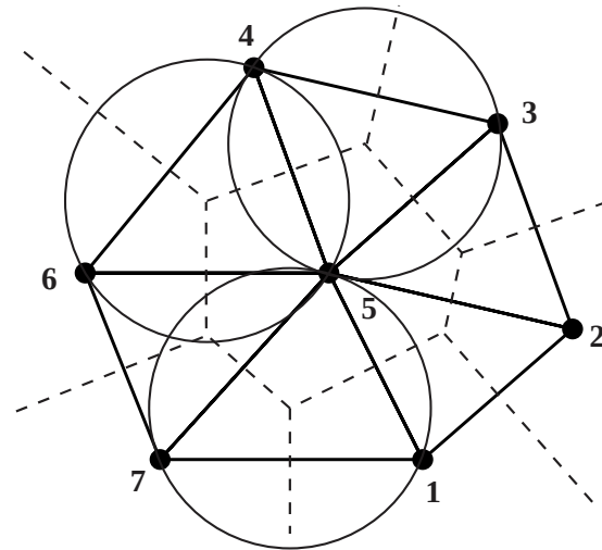
شکل 3 مثلث‌بندی دلانی برای گره
