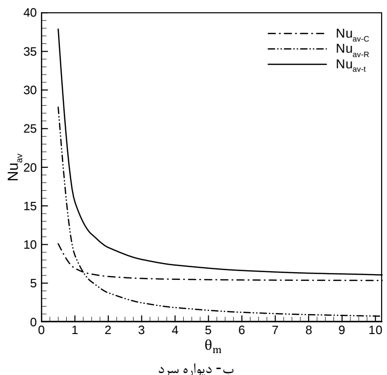
شکل 15 تغییرات عدد ناسلت متوسط برحسب دمای متوسط بدون بعد
