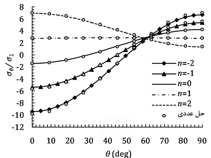
شکل 14 توزیع تنش محیطی در اطراف گشودگی ورق ناهمگن با روند کاهشی مدول الاستیسیته بدون فشار (کشش دوماحوری)
