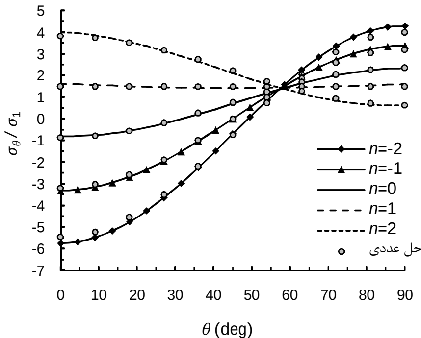
شکل 16 توزیع تنش محیطی در اطراف گشودگی ورق ناهمگن با روند افزایشی مدول الاستیسیته بدون فشار (کشش دوماحوری)
