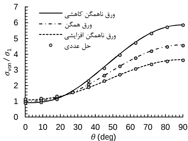
شکل 5 توزیع تنش فون میزز در اطراف گشودگی تحت فشار یکنواخت (کشش تک محوری)
