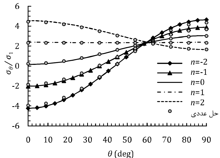
شکل 17 توزیع تنش محیطی در اطراف گشودگی ورق ناهمگن با روند افزایشی مدول الاستیسیته تحت فشار یکنواخت (کشش دوماحوری)
