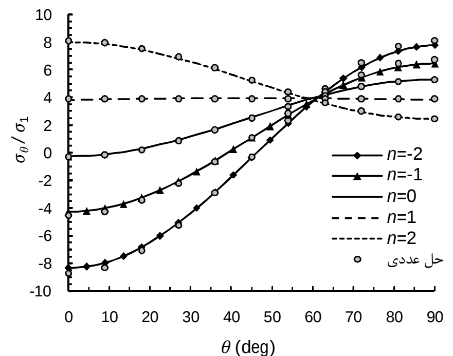
شکل 15 توزیع تنش محیطی در اطراف گشودگی ورق ناهمگن با روند کاهشی مدول الاستیسیته تحت فشار یکنواخت (کشش دوماحوری)
