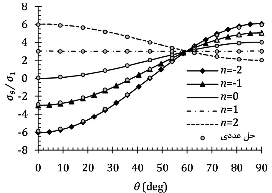
شکل 13 توزیع تنش محیطی در اطراف گشودگی ورق همگن تحت فشار یکنواخت (کشش دوماحوری)
