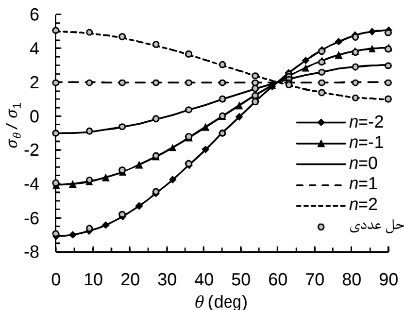
شکل 12 توزیع تنش محیطی در اطراف گشودگی ورق همگن بدون فشار (کشش دوماحوری)
