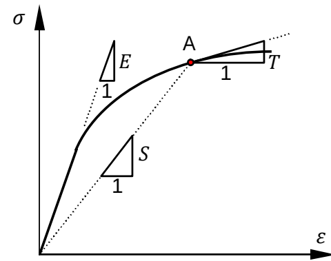
شکل 2 نمایش طرح‌واره مدول الاستیسیته، مدول مماسی و مدول وتري در نقطه دلخواه A از منحنی تنش- کرنش
