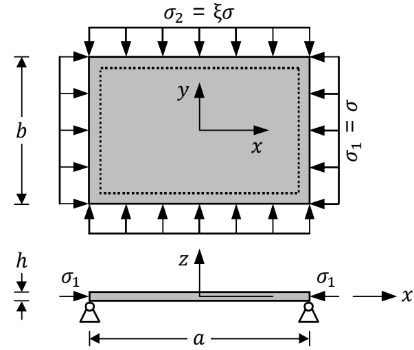
شکل 1 نمایش طرح‌واره هندسه و بارگذاری صفحه مستطیلی، تحت بارگذاری دومحوره با نسبت بارگذاری \xi و تکیه‌گاه ساده در چهار لبه
