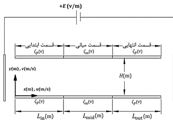
شکل 3 مشخصات ریزمجرای ناهمگن مورد بررسی و محورهای مختصات
