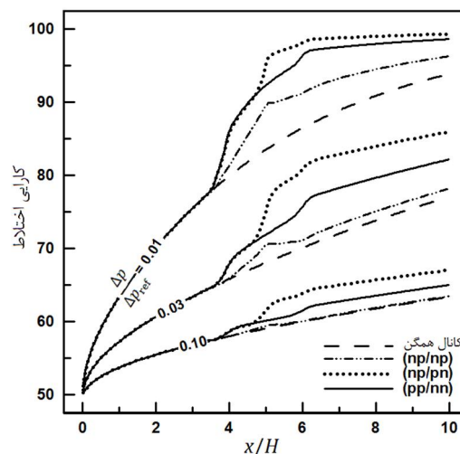
شکل 8 تغییرات راندمان اختلاط در طول ریزمجرا برای اختلاف فشارهای مختلف و آرایش‌های متفاوت تکه‌های ناهمگنی بار
