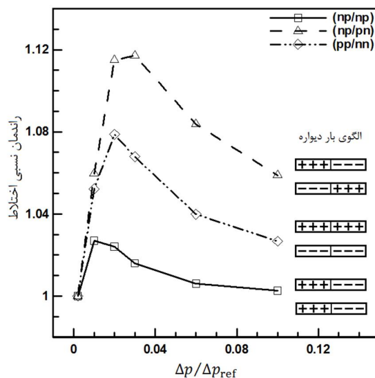
شکل 10 تغییرات راندمان نسبی اختلاط، E_{\text{chr}} ، به‌ازای تغییرات اختلاف فشار \Delta p برای سه آرایش بار مختلف
