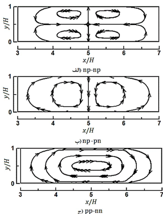
شکل 6 جریان الکترواسموتیک برای سه آرایش متفاوت بارهای قسمت میانی الف- np-np ب- np-pn ج- pp-nn
