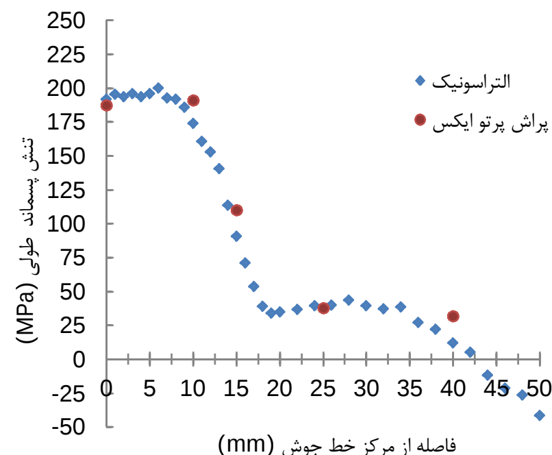
شکل 10 تنش پسماند طولی اندازه گیری شده با دو
