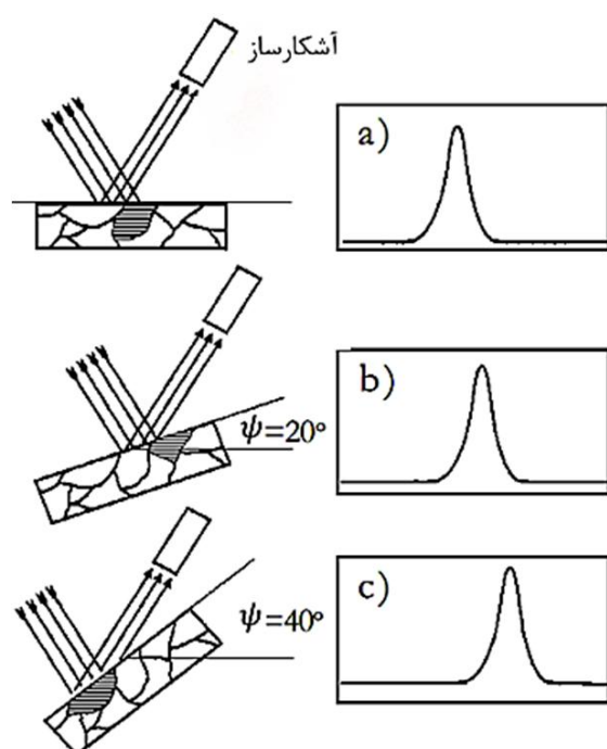
شکل 13 شیب دادن به قطعه در برابر پرتو و جابه جایی پیک پراش [22]
