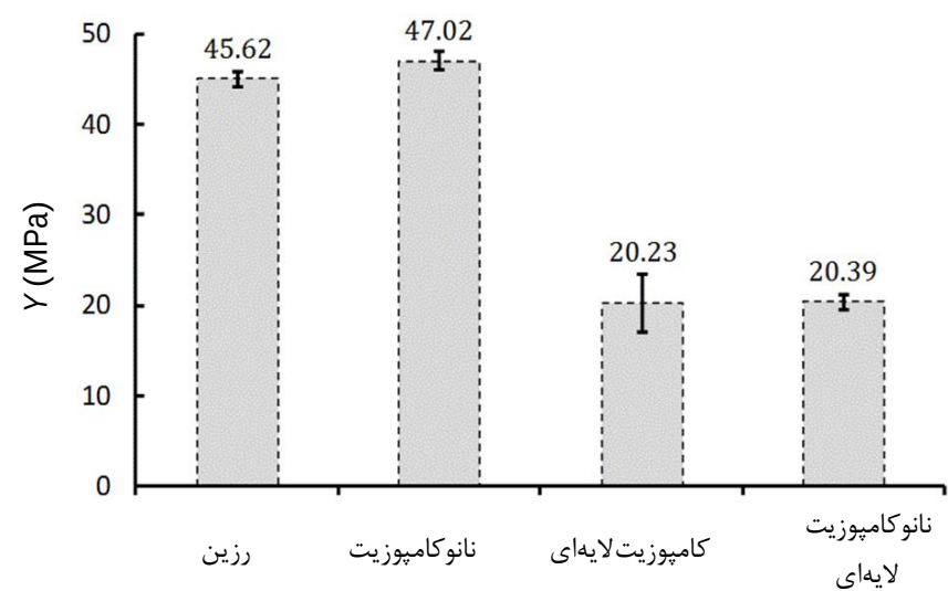
شکل 14 مقایسه مقدار Y_T برای چهار ماده مختلف
