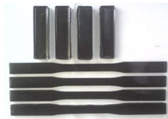
شکل 5 نمونه‌های استفاده‌شده برای انجام آزمایش‌های مکانیکی نانوکامپوزیت
