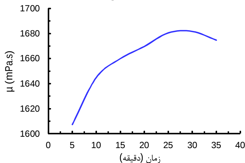
شکل 4 نمودار تغییرات گرانیوی برحسب زمان انرژی‌دهی مافوق صوت برای 0/5 درصد وزنی نانولوله کربنی چند جداره
