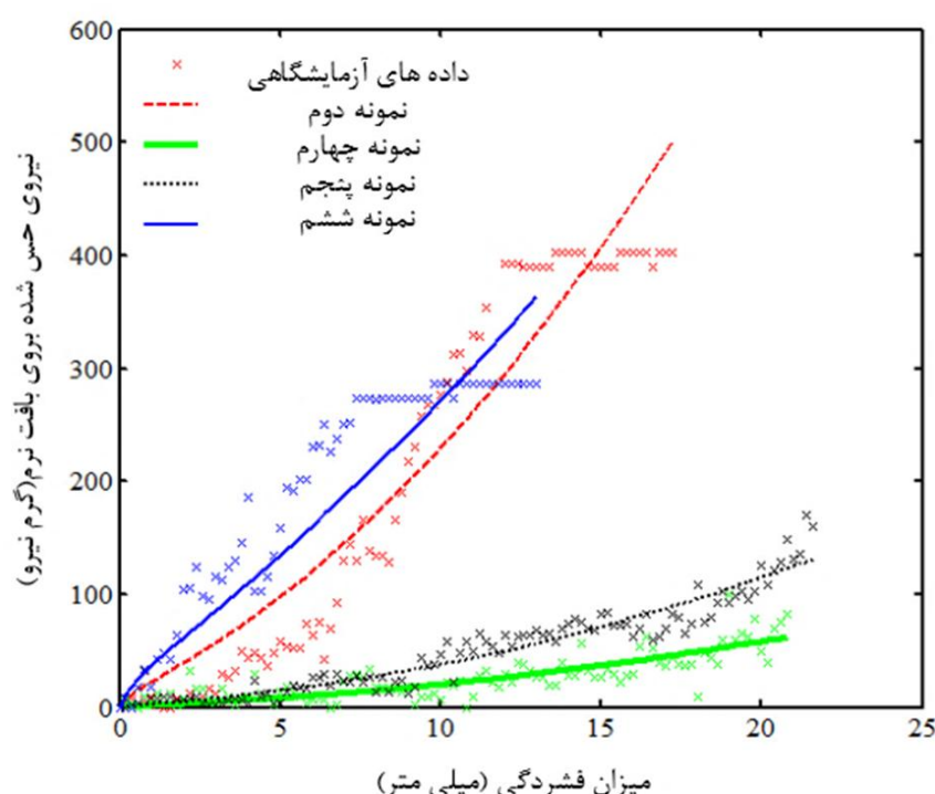
شکل 8 بررسی نقطه‌ی متناظر ساعت 8 بین چهار نمونه از افراد معاینه شده توسط دستگاه
