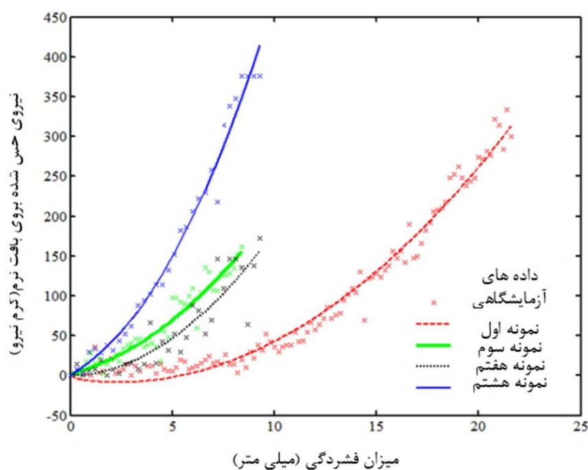
شکل 9 بررسی نقطه‌ی متناظر ساعت 9 بین چهار نمونه از افراد معاینه شده توسط دستگاه
