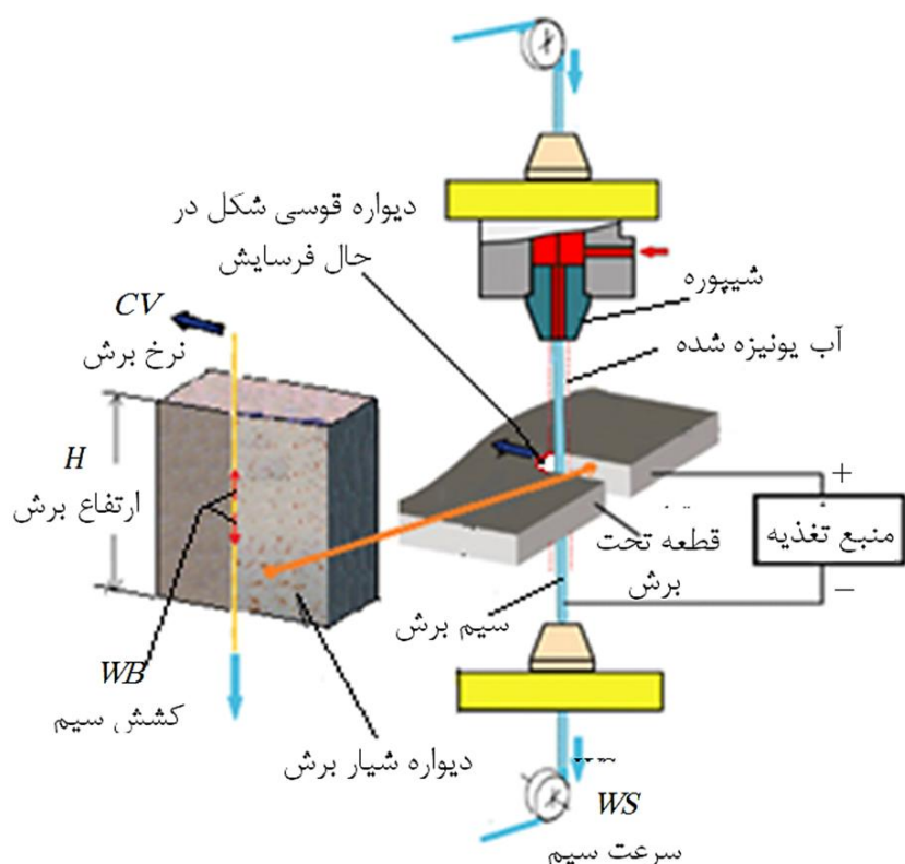
شکل 1 نمایشی از عمل برش سیمی قطعه به روش تخلیه الکتریکی
