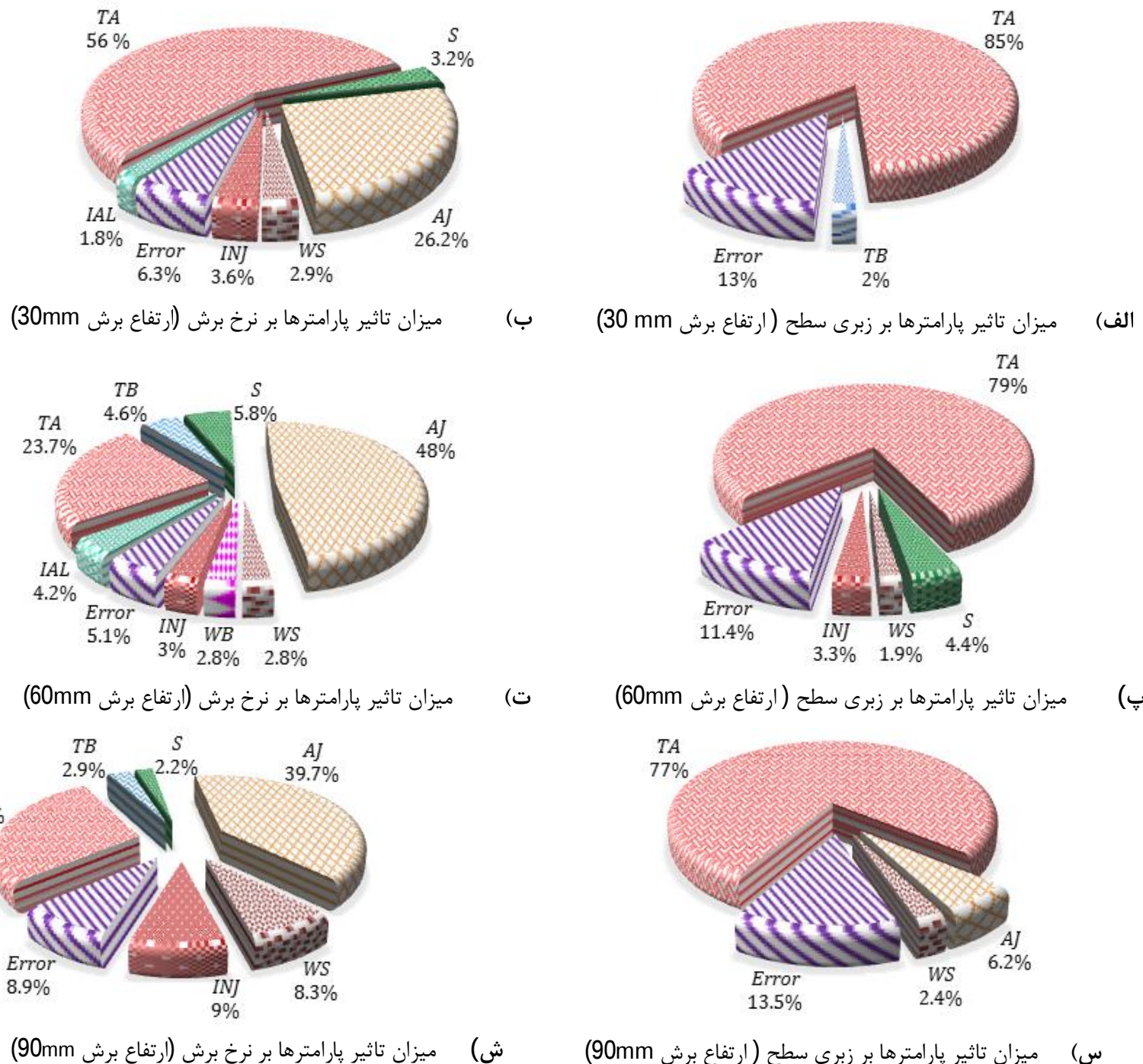
شکل 6 میزان مشارکت پارامترهای معنی دار شناسایی شده با آنالیز واریانس بر نرخ برش و زبری سطح قطعات تیتانیومی برش خورده در سه ارتفاع 30، 60، 90 mm
