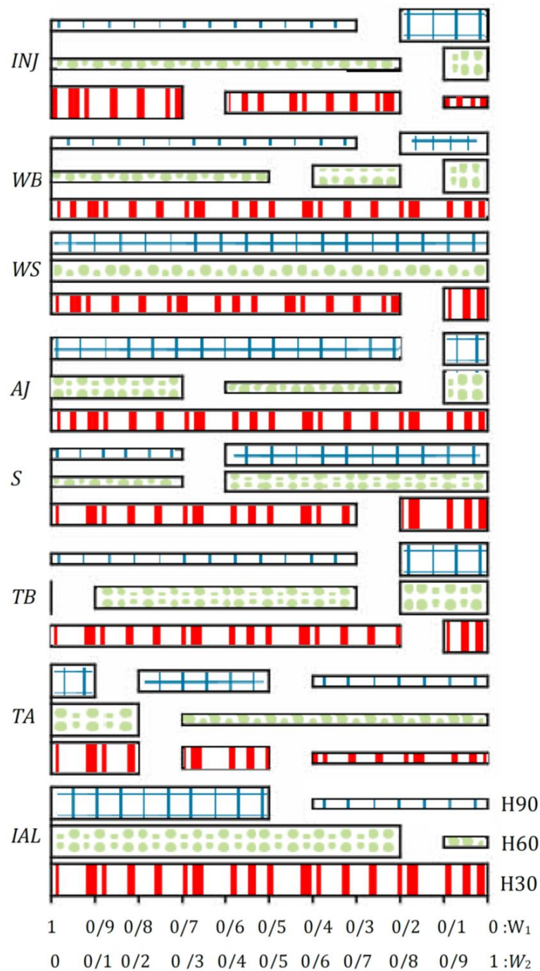
شکل 7 مقدار بهینه پارامترها برحسب تغییر ضرایب اهمیت نرخ برش و زبری سطح، برای سه ارتفاع برش 30، 60، 90 میلی متر برای هر 3 ارتفاع برش (30، 60 و 90mm) از میان 8 پارامتر مورد بررسی، پارامتر زمان روشنی پالس (TA) بدلیل تاثیر بیش از 77٪، اثرگذارترین پارامتر بر زبری سطح و دو پارامتر TA و ولتاژ متوسط ماشین کاری (AJ) با مجموع تاثیر بیش از 67/5٪ پارامترهای پر اثر بر نرخ برش ماشین کاری آلیاژ تیتانیوم معرفی می شوند. (ارجاع به شکل 6)
