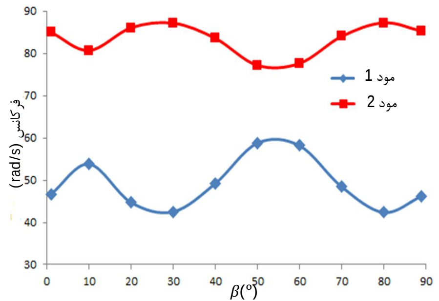
شکل 16 تغییرات فرکانس‌های طبیعی مود اول و دوم ملخ برحسب زاویه گام در حالت دورانی
