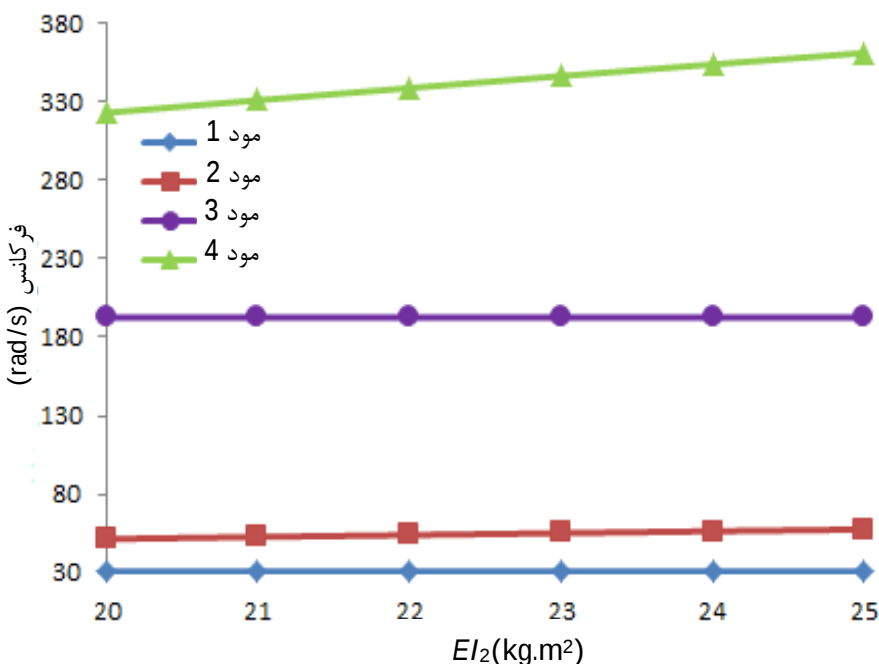
شکل 10 تغییرات فرکانس‌های طبیعی ملخ برحسب سختی خارج از صفحه دوران
