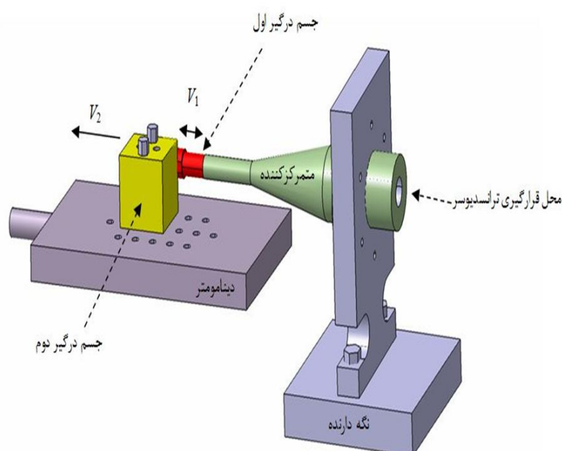
شکل 7 شماتیک درگیری جسم اول و دوم
