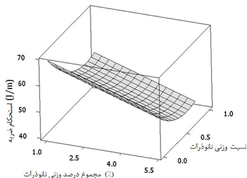
شکل 7 روبه پاسخ استحکام ضربه، مقدار ثابت: درصد وزنی PP-MA
