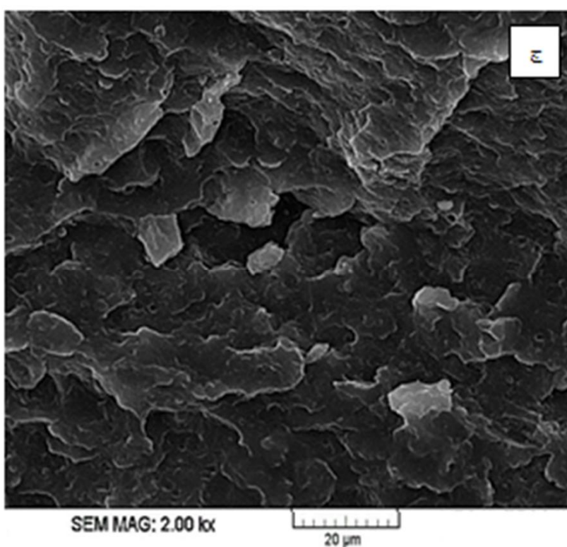
شکل 2 ریزنگارهای SEM گرفته شده از ترکیبات پلی پروپیلن پر شده با گرافن و نانورس با بزرگنمایی 2000 برابر:
