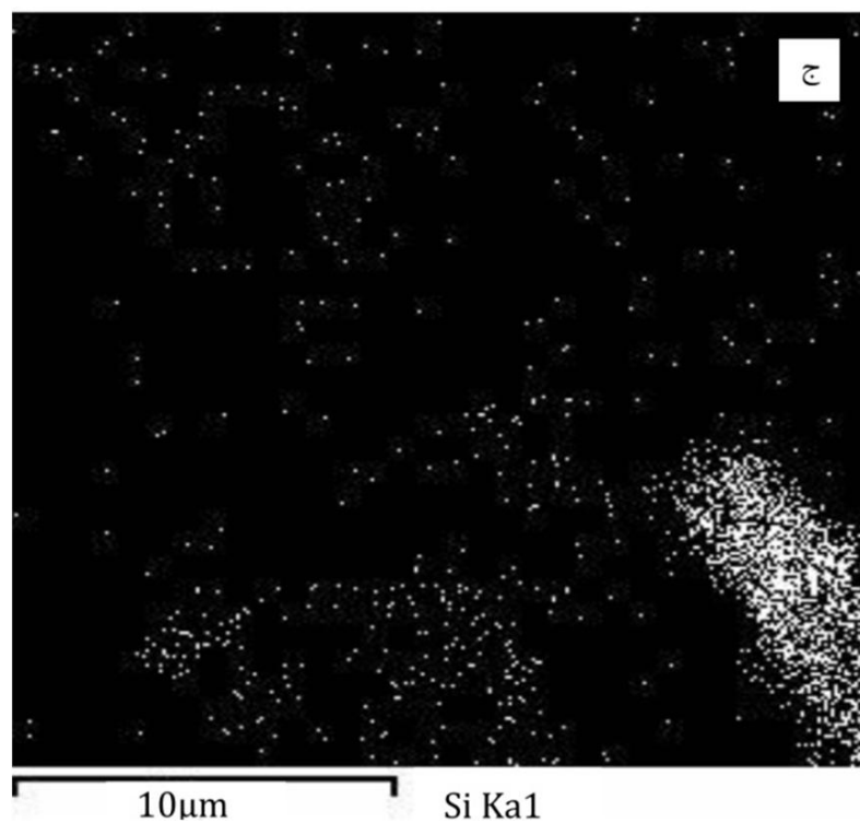
شکل 3 ریزنگارهای SEM گرفته شده همراه با EDX از ترکیبات پلی پروپیلن پر شده با گرافن و نانورس: (الف) 97PP/0.5G/0.5C/2PP-MA (ب) 95PP/1G/2C/2PP-MA (ج) 93PP/2.5G/2.5C/2PP-MA
