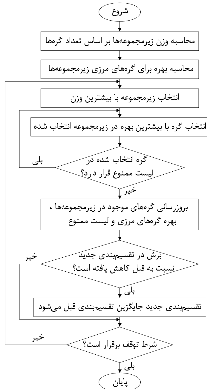
شکل 4 فلوچارت الگوریتم جستجوی ممنوع برای تقسیم‌بندی گراف
