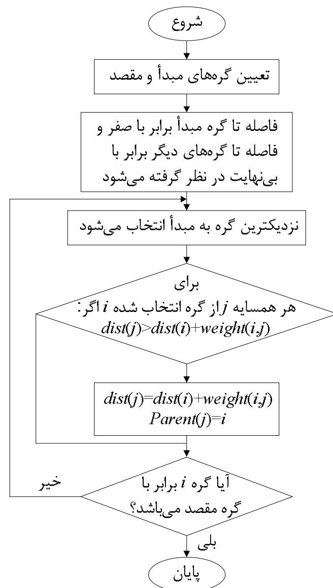
شکل 6 فلوچارت الگوریتم کوتاهترین مسیر برای تولید شبکه درشت دوگانه
