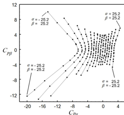
شکل 8 منحنی کالیبراسیون پراب پنج حفره برای ضرایب فشار زاویه پیچ و یو
