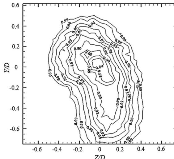
شکل 10 توزیع نسبت سرعت (U/U_\infty) در مقطع X/L=0/85 پشت مدل سابوف
