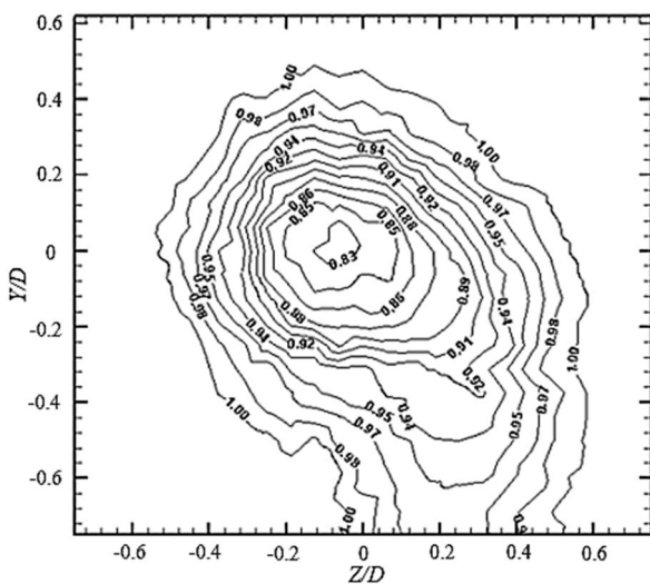
شکل 26 توزیع نسبت سرعت ( U/U_\infty ) در فاصله X/L=1 پشت مدل زیردریایی تانگو
