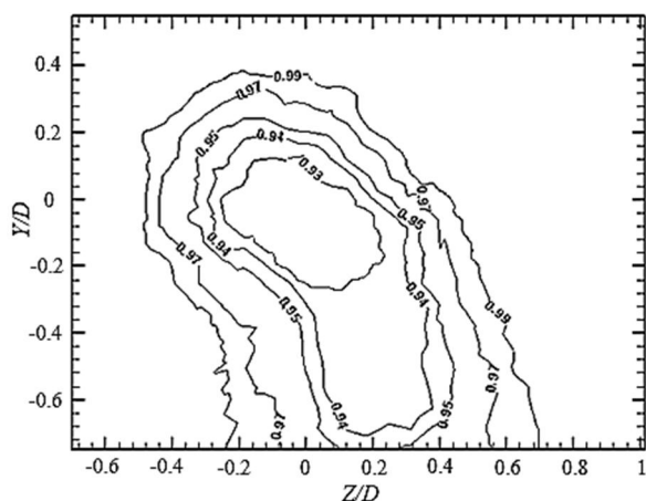
شکل 13 توزیع نسبت سرعت (U/U_\infty) در فاصله X/L=1/5 پشت مدل سابوف
