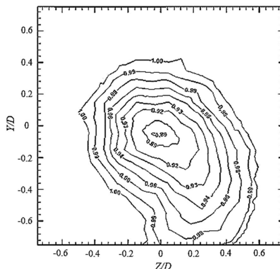
شکل 11 توزیع نسبت سرعت (U/U_\infty) در فاصله X/L=1 پشت مدل سابوف
