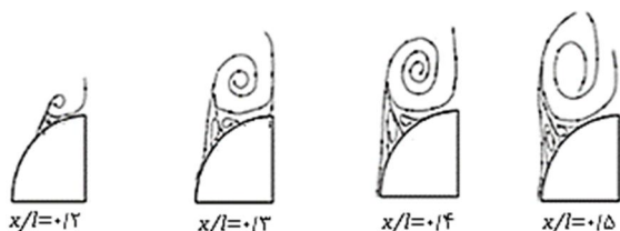
شکل 16 ساختار گردابه‌ها در پژوهش سعیدی‌نژاد و همکاران [16]
