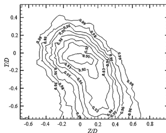
شکل 12 توزیع نسبت سرعت (U/U_\infty) در فاصله X/L=1/25 پشت مدل سابوف
