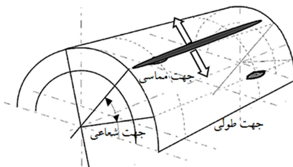
شکل 19 ایجاد ترک‌های طولی در سطح خارجی لوله‌های تولید شده با فرآیند پیلگر سه غلتکه [11]
