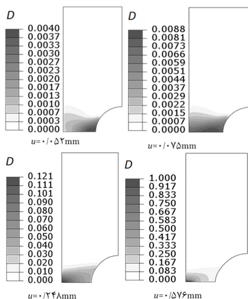
شکل 3 کانتور توزیع آسیب پیش‌بینی شده توسط دو معیار کمتر و کمتر اصلاح شده در میله شیاردار استوانه‌ای در کشش‌های مختلف
