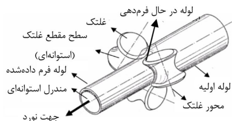
شکل 1 شماتیک فرآیند نورد پیلگر به روش سه‌غلته
