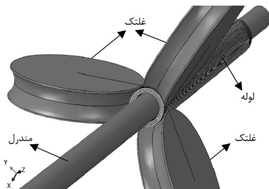
شکل 11 مدل کامل فرآیند پیلگر سه غلتک بدون استفاده از تقارن
