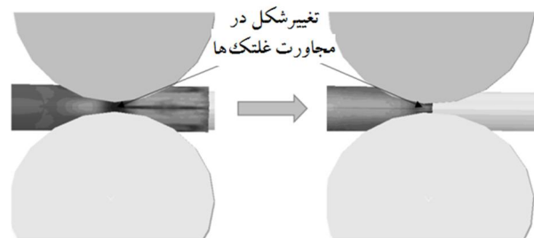
شکل 18 تغییر شکل نقاط مجاور غلتک‌ها در لوله
