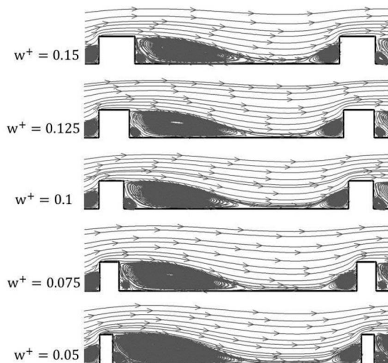
شکل 14 خطوط جریان کانال زیر مستطیلی با ارتفاع بی‌بعد ثابت h^+ = 0.1 برای عرض‌های مختلف بی‌بعد زبری
