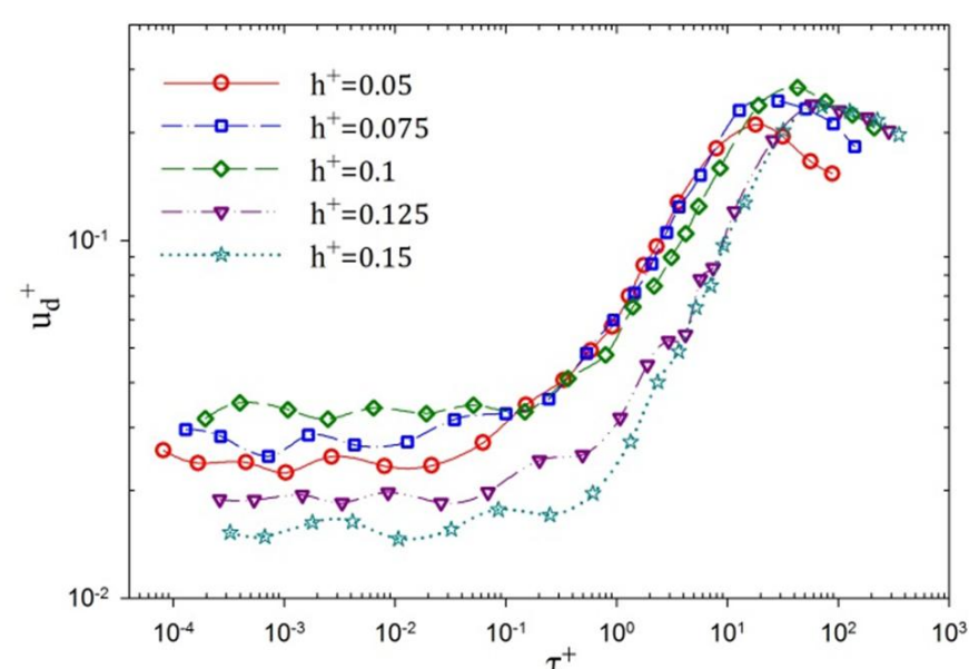
شکل 13 تغییرات سرعت رسوب بی‌بعد برای کانال زیر مستطیلی عمودی با عرض بی‌بعد ثابت w^+ = 0.1 برای ارتفاع‌های بی‌بعد مختلف زبری با گرانش در جهت جریان
