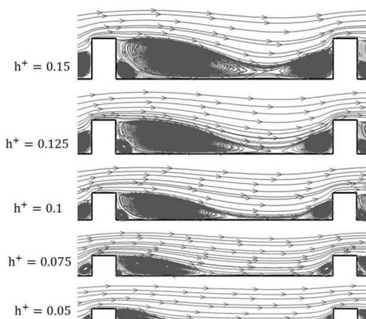
شکل 11 خطوط جریان کانال زیر مستطیلی با عرض بی‌بعد ثابت w^+ = 0.1 برای ارتفاع‌های مختلف بی‌بعد زبری
