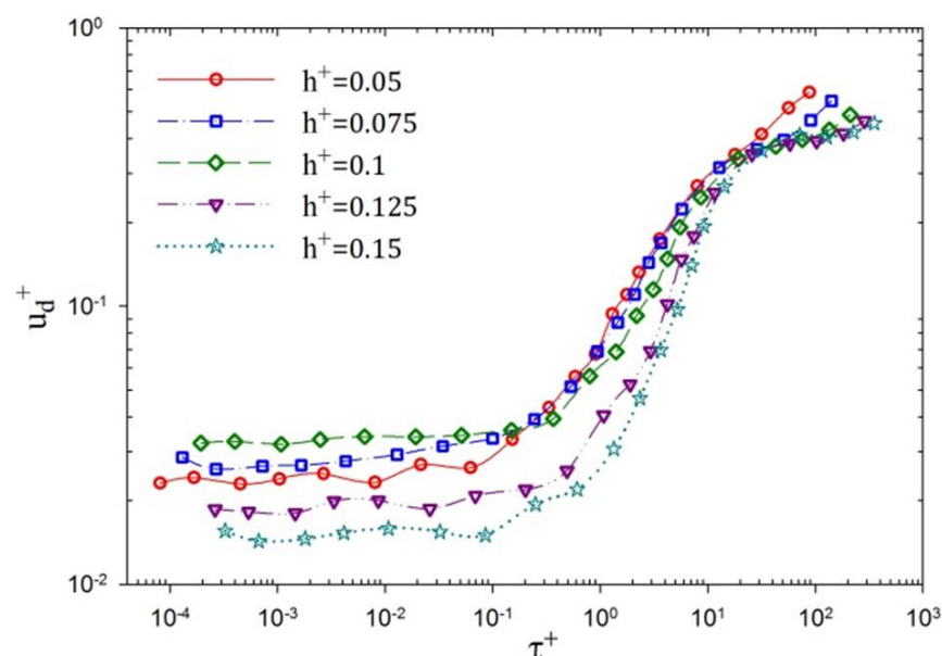
شکل 12 تغییرات سرعت رسوب بی‌بعد برای کانال زیر مستطیلی افقی با عرض بی‌بعد ثابت w^+ = 0.1 برای ارتفاع‌های بی‌بعد مختلف زبری با گرانش عمود بر جهت جریان
