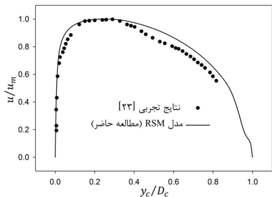
شکل 3 پروفیل بی‌بعد سرعت متوسط جریان اصلی در جریان توسعه یافته کانال نامتقارن
