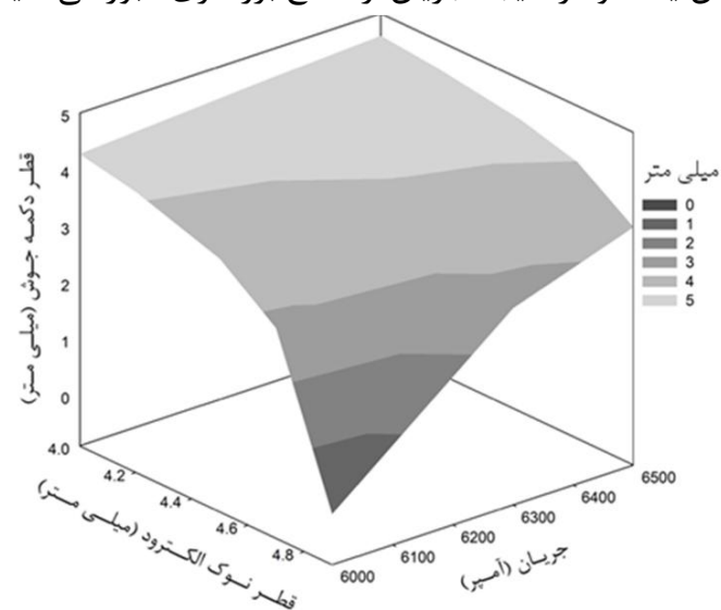
شکل 7 تأثیر همزمان جریان جوشکاری و قطر نوک الکترود بر قطر دکمه جوش
