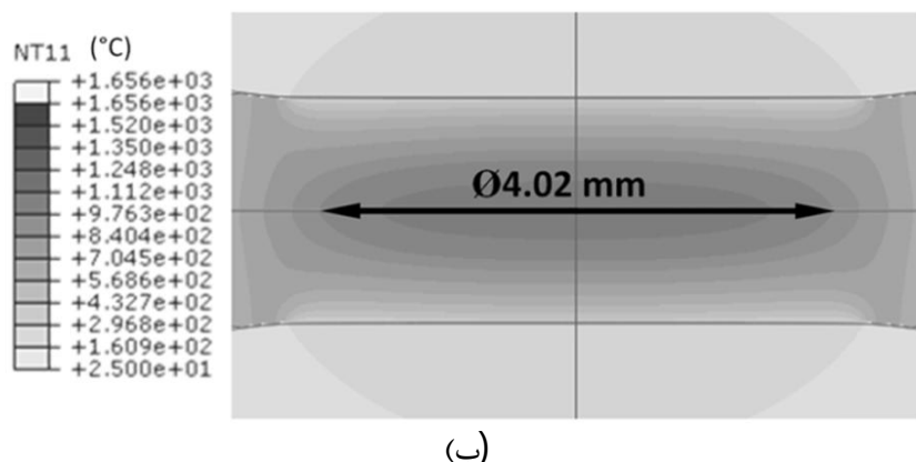
شکل 4 مقایسه نتایج بدست آمده از (الف) آزمایش‌های تجربی و (ب) شبیه‌سازی حرارتی برای جریان 6/5 کیلو آمپر و مدت زمان جوشکاری 10 سیکل
