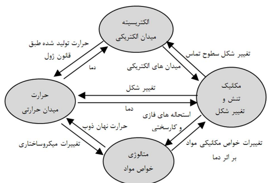
شکل 1 تأثیر حوزه‌های مختلف بر یکدیگر در فرایند جوشکاری مقاومتی
