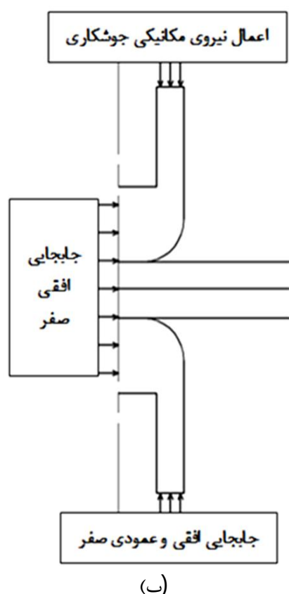
شکل 3 شرایط مرزی استفاده شده در فرایند تحلیل (الف) حرارتی-الکتریکی و (ب) تحلیل مکانیکی
