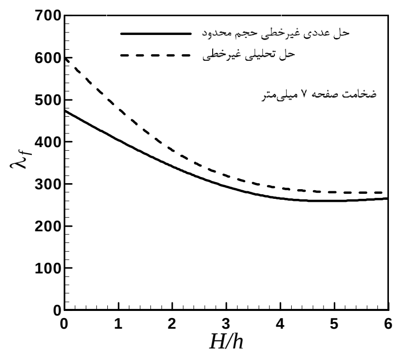
شکل 15 مقایسه فشار دینامیکی فلاتر بی‌بعد برحسب انحنای پوسته به دو روش عددی و تحلیلی
