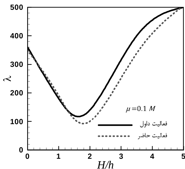
شکل 17 مقایسه نتایج فشار دینامیکی فلاتر صفحه برحسب انحنا با مرجع [24]
