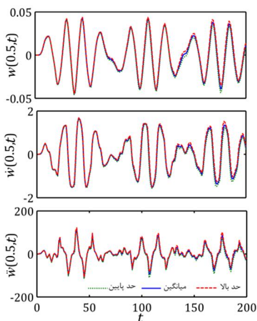
شکل 14 پاسخ‌های دینامیکی لوله حامل جریان چندفازی براساس مدل غیرخطی
