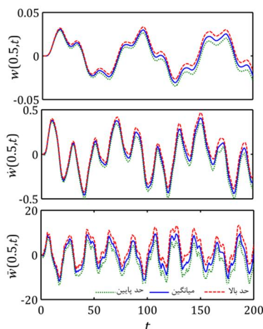
شکل 7 پاسخ‌های دینامیکی لوله حامل جریان چندفازی به‌ازای U = 1/5 و A = 3
