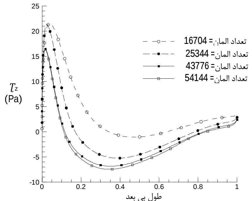
شکل 8 توزیع مولفه محوری تنش برشی دیواره پایینی مجرای خم 90 درجه برای چهار اندازه شبکه مختلف
