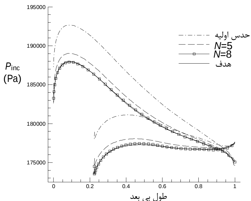
شکل 11 روند همگرایی توزیع فشار افزایش یافته
