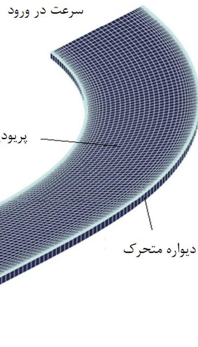
شکل ۷ شرایط مرزی مجرای خم ۹۰ درجه
