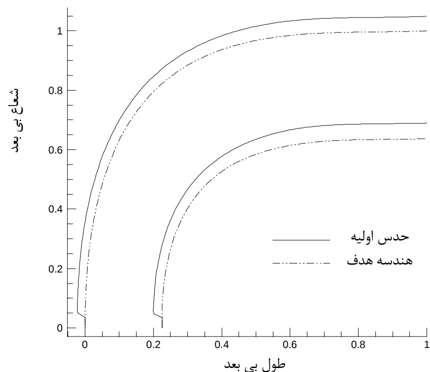
شکل 14 هندسه حدس اولیه با ناپیوستگی
