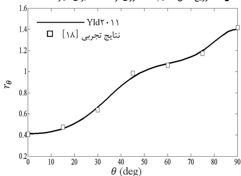
شکل 13 توزیع تنش تسلیم تک‌محوری نرماله شده برای آلیاژ AA3104-H19
