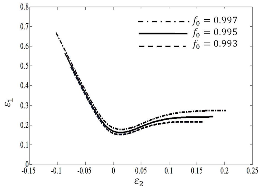
شکل 8 اثر ضریب نقص اولیه بر FLC براساس معیار تسلیم Yld2011
