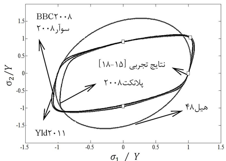
شکل 2 سطح تسلیم پیش‌بینی شده برای آلیاژ AA2090-T3
