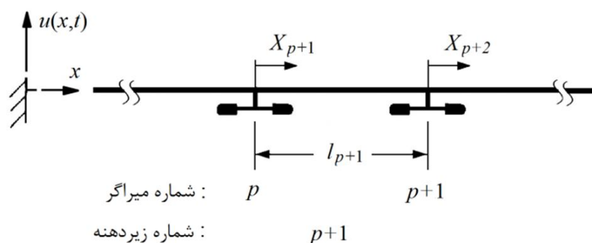
شکل 7 کابل دارای بیش از یک میراگر
