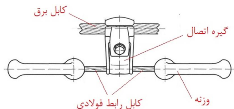
شکل 1 میراگر استاکبریج [3]
