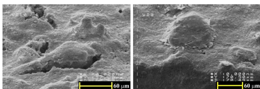
شکل 5 تصویر میکروسکوپ الکترونی روبشی سطح نمونه 2 با زاویه 45 درجه و با بزرگ‌نمایی 10000 برابر - نمونه‌ای از ترک‌ها و تپه‌ها بر روی سطح
