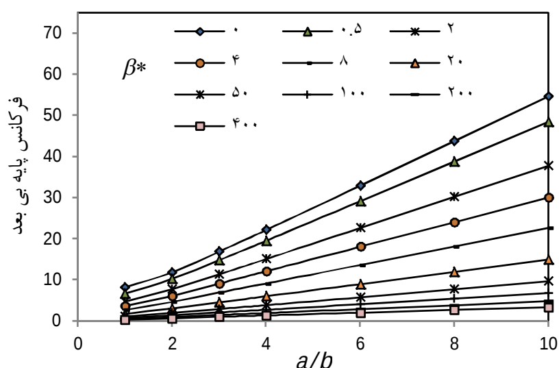
شکل 3 تأثیرات نسبت ابعادی بر اولین فرکانس طبیعی بی بعد نانوورق با چهار تکیه‌گاه گیردار برای پارامترهای غیرمحلی بی بعد مختلف \nu = 0/3 و b = 5h
