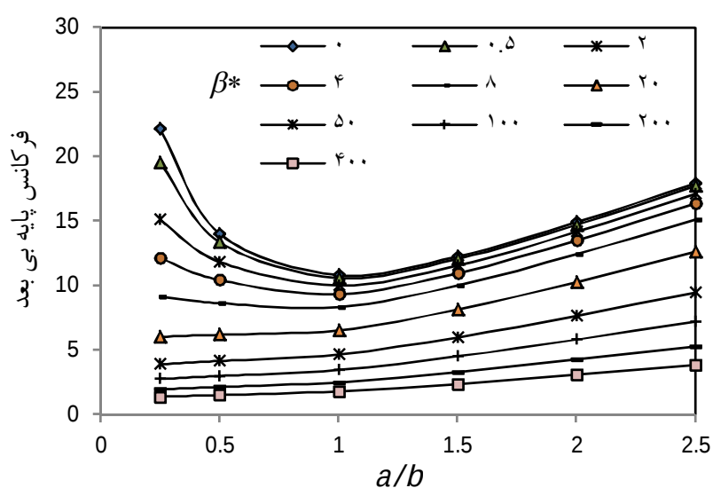
شکل 4 تأثیرات نسبت ابعادی بر اولین فرکانس طبیعی بی بعد نانوورق با چهار تکیه‌گاه گیردار برای پارامترهای غیرمحلی بی بعد مختلف \nu = 0/3 و b = 20h
