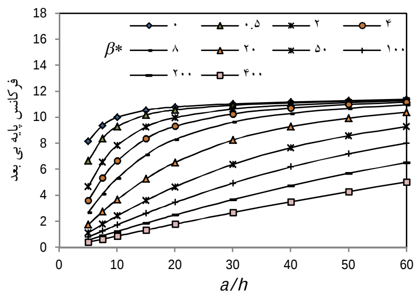
شکل 2 تأثیر نسبت طول به ضخامت بر اولین فرکانس طبیعی بی بعد نانوورق مربعی با چهار تکیه‌گاه گیردار برای پارامترهای غیرمحلی بی بعد مختلف \nu = 0/3
