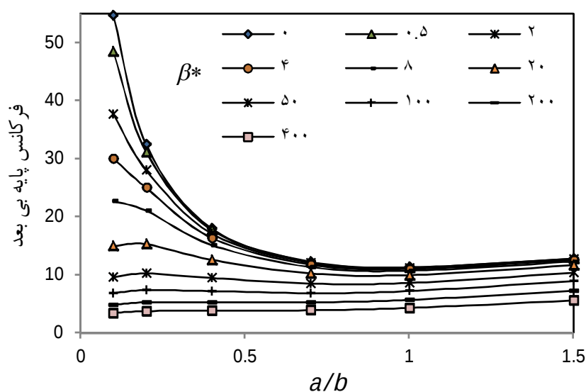
شکل 5 تأثیرات نسبت ابعادی بر اولین فرکانس طبیعی بی بعد نانوورق با چهار تکیه‌گاه گیردار برای پارامترهای غیرمحلی بی بعد مختلف \nu = 0/3 و b = 50h
