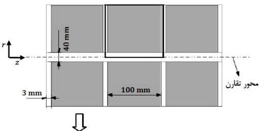
شکل 1 هندسه کلی مخزن هیدرید فلزی در نظر گرفته شده
