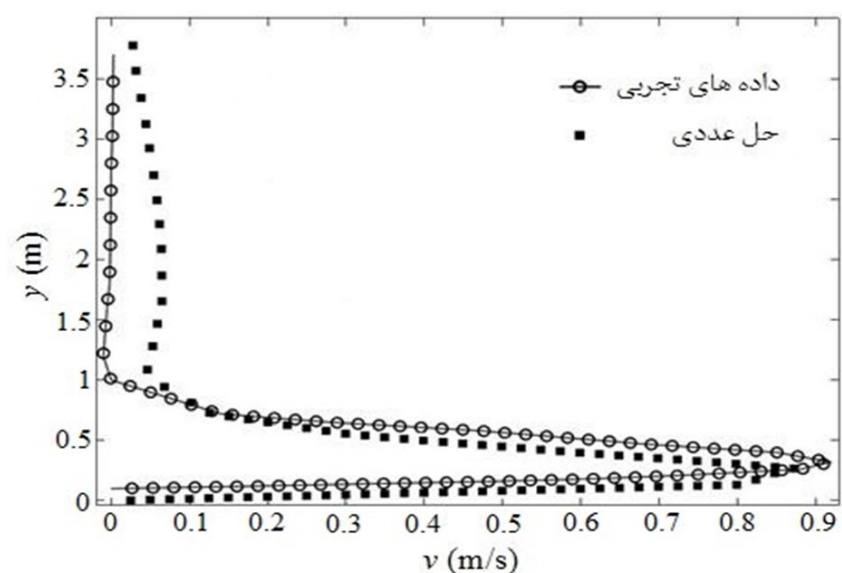
شکل 8 پروفیل‌های سرعت حاصل از حل عددی و کار تجربی سنسناک‌ریشن
