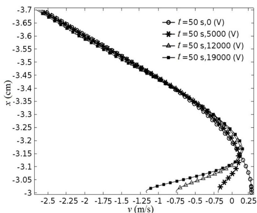
شکل 16 پروفیل مؤلفه‌ی سرعت در جهت y (V) در عدد رینولدز 6000 در نقطه‌ی y = -1/22 (ناحیه‌ی بین دو الکتروده)
