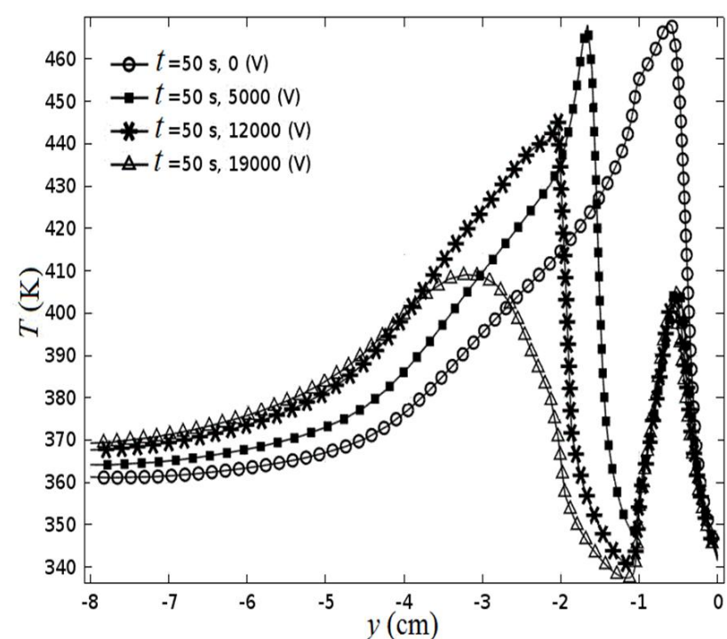
شکل 23 نمودار دمای سطح لوله در قسمت قرارگیری محرک، رینولدز 4500
