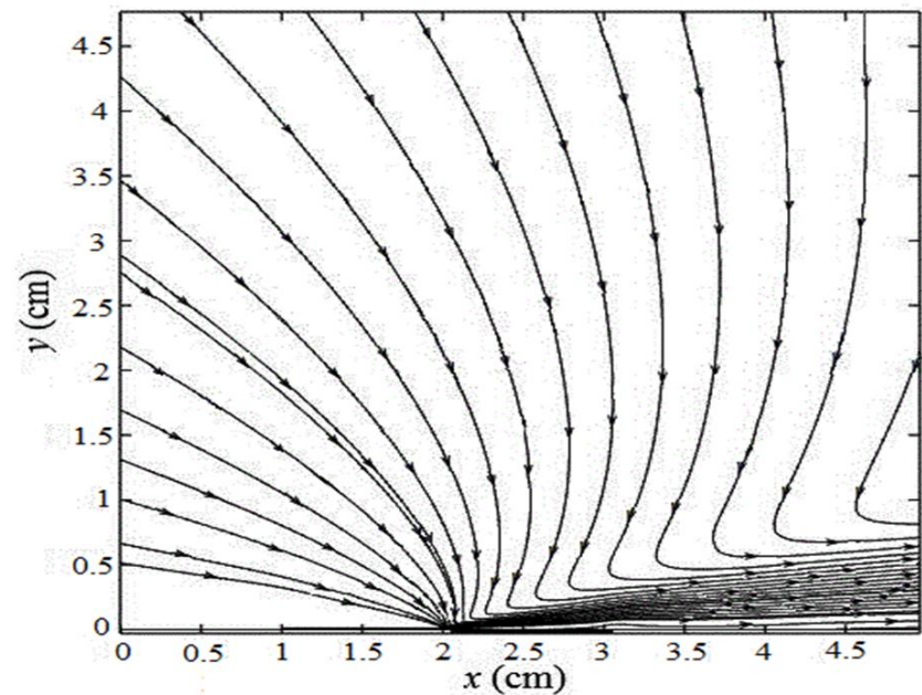
شکل 7 خطوط جریان حاصل از کار شبیه‌سازی ما، ماکزیمم سرعت 1 m/s
