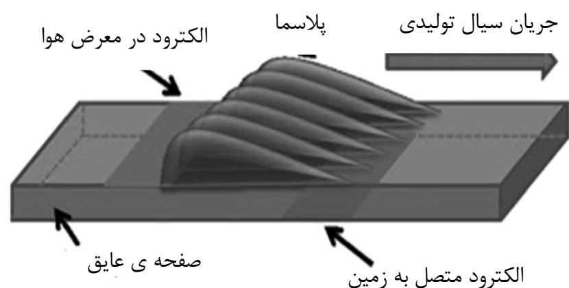
شکل 1 نمایی کلی از یک تک محرک DBD مسطح
