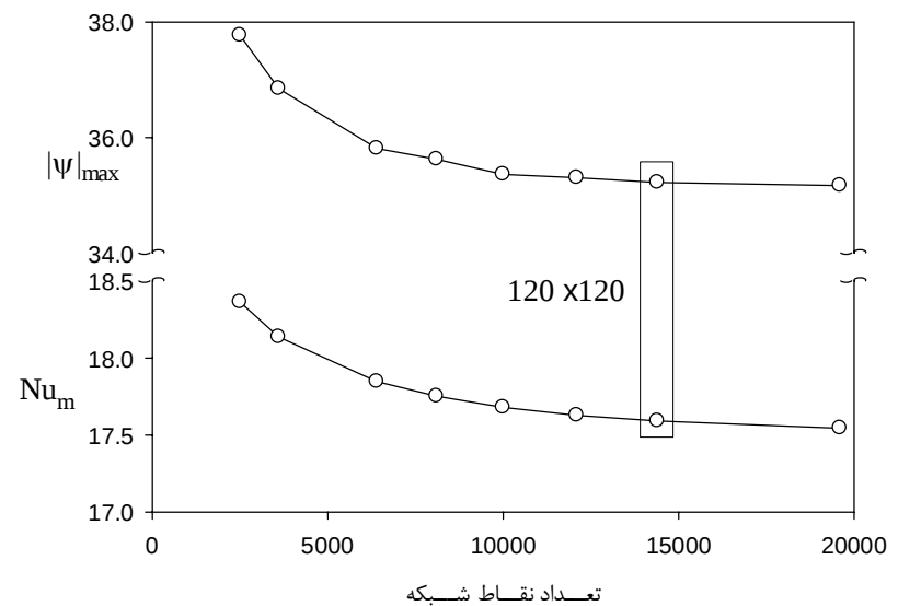
شکل 3 تأثیر تعداد نقاط شبکه بر روی عدد نوسلت متوسط دیوار سرد و بیشترین مقدار تابع جریان ( Ra = 10^6, n = 0.8, B = 0.2, D = 0.3 )
