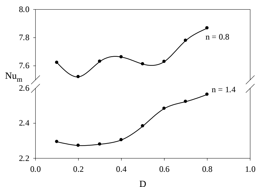
شکل 15 تغییرات عدد نوسلت متوسط بر حسب فاصله‌ی مانع‌ها از یکدیگر در n = 0.8, 1.4 ، ( Ra = 10^5, B = 0.2 )
