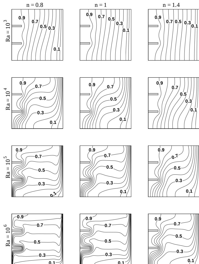
شکل 6 خطوط هم‌دما در اعداد رایی و شاخص تابع نمایی مختلف ( B = 0.2, D = 0.3 )
