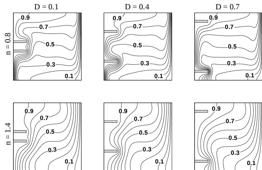
شکل 14 خطوط هم‌دما در سه موقعیت مختلف برای مانع‌ها و در n = 0.8 (بالا) و n = 1.4 (پایین)، ( Ra = 10^5, B = 0.2 )
