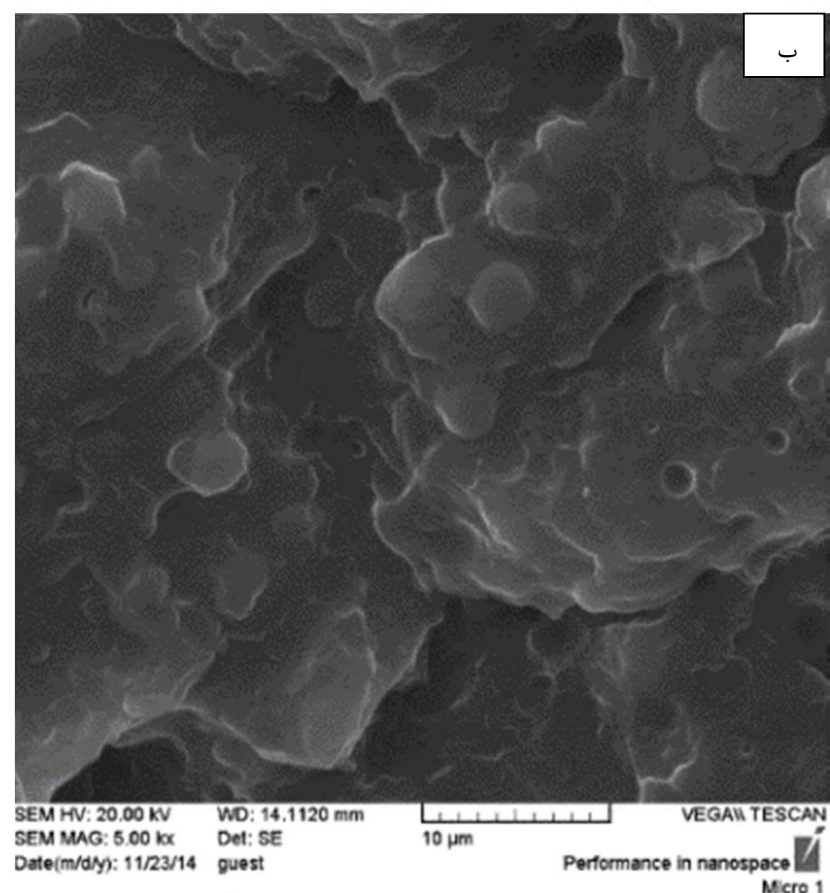
شکل 6: تصاویر SEM با بزرگنمایی 5000x برای نمونه‌های (الف 30E16T و ب 15E8T)
