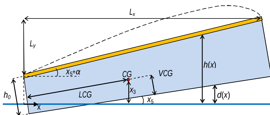
شکل 4 تعاریف هندسی مربوط به مدل آیرودینامیکی
