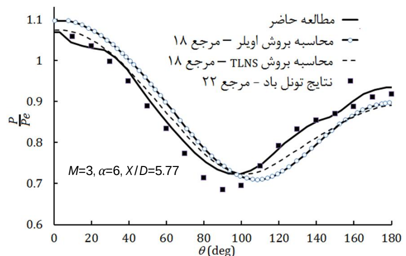
شکل 5 توزیع فشار محیطی در مقطع X/D=5.77
