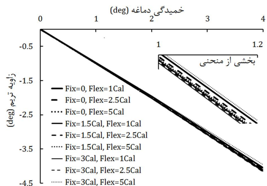
شکل 20 منحنی‌های تریم در ماخ 5
