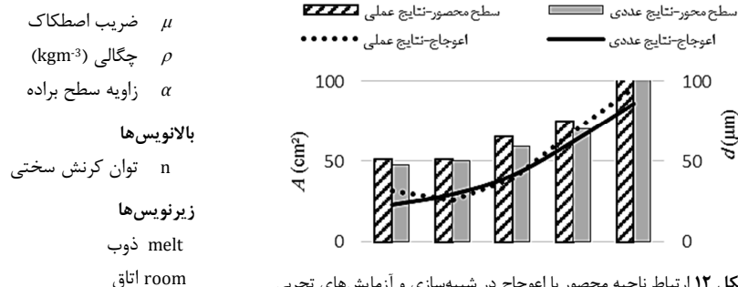
شکل ۱۲ ارتباط ناحیه محصور با اعوجاج در شبیه‌سازی و آزمایش‌های تجربی
