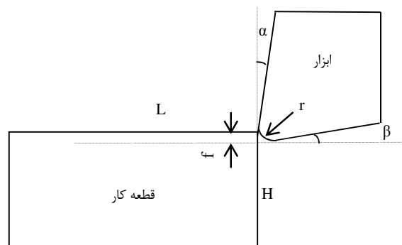
شکل ۳ مدل هندسی شبیه‌سازی و پارامترهای ابعادی مؤثر
