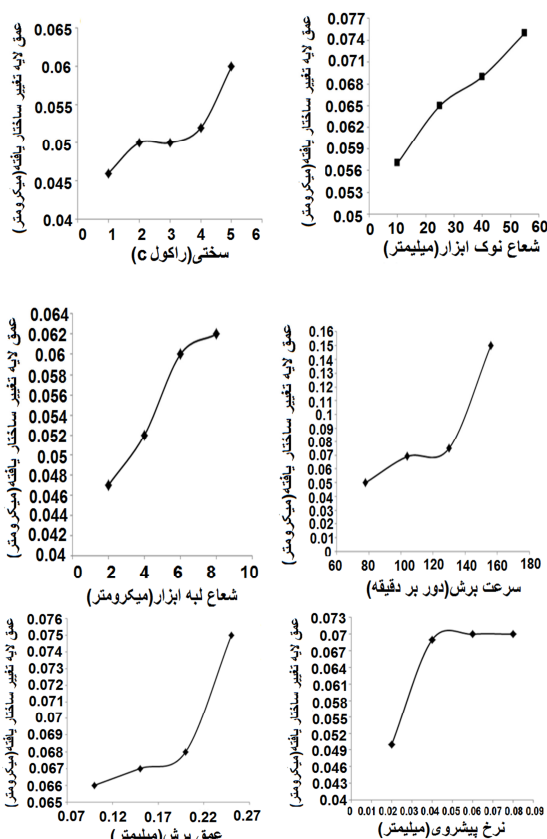
شکل ۱۱ نمودار اثر تغییر سختی قطعه‌کار (مدل ماده)، نرخ پیشروی ابزار، تغییر شعاع لبه ابزار و شعاع نوک ابزار و سرعت برش در تغییرات عمق لایه تغییر شکل یافته در شبیه‌سازی فرآیند ماشین‌کاری
