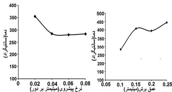
شکل ۴ اثر پارامترهای ماشین کاری بر دمای قطعه
