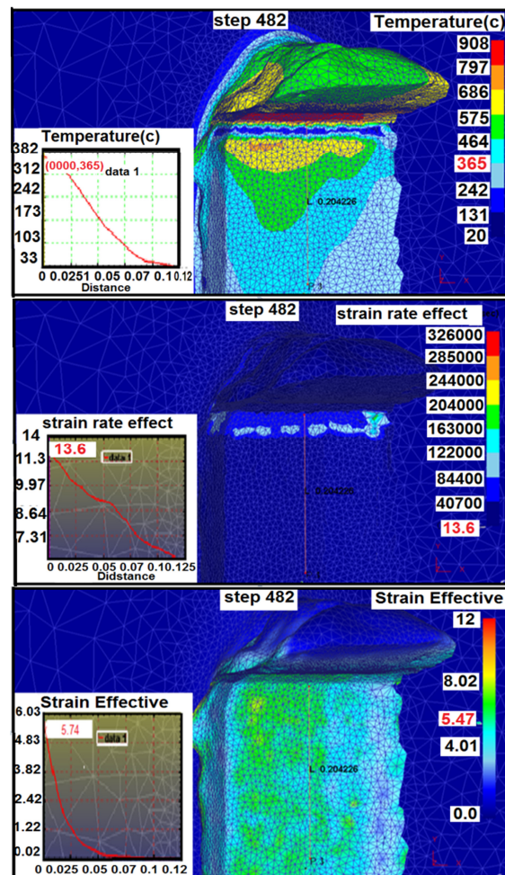
شکل ۹ نحوه اندازه‌گیری دما و نرخ کرنش و نرخ کرنش موثر جهت رسم نمودار تغییر کرنش مکانیکی در عمق قطعه‌کار در شبیه‌سازی با فاصله ۰/۲ میلی‌متر از لبه براده
