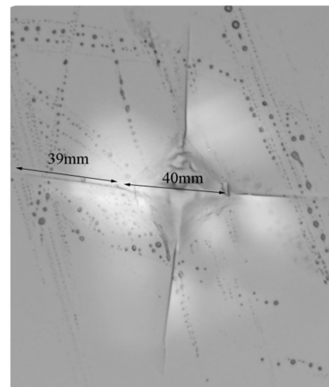
شکل ۲ اثر نوک ویکرز بر روی شیشه BK7 در اثر نیروی ۵۰۰ گرمی
