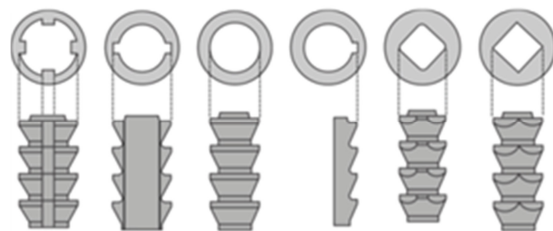
شکل ۱ نمونه‌هایی از پروفیل‌های جلویی ابزارهای خان‌کشی [۸]
