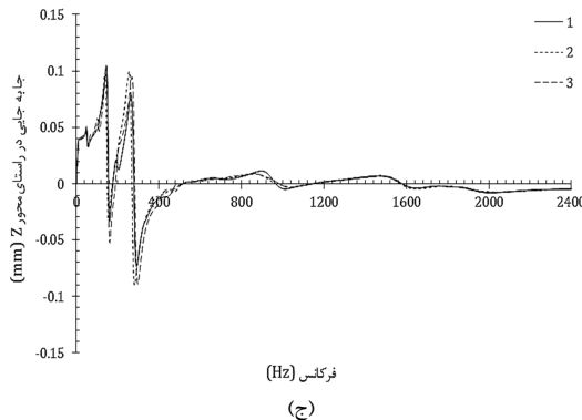
شکل ۶ جابه‌جایی نوک ابزار در حالت هارمونیک برای وضعیت‌های قرارگیری اسپیندل در موقعیت‌های ۱، ۲ و ۳
