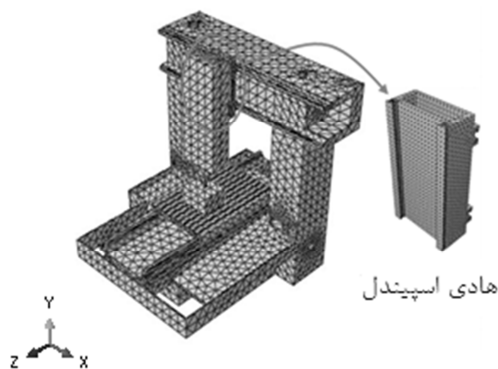
شکل ۲ مدل مش‌بندی شده دستگاه
