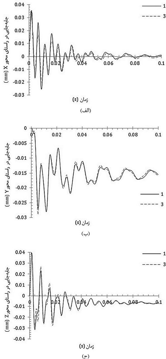
شکل ۴ جابه‌جایی نوک ابزار در حالت گذار برای دو وضعیت قرارگیری اسپیندل
