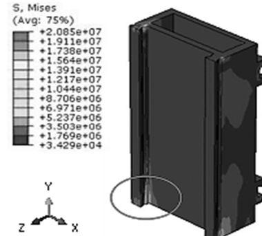
شکل ۵ موقعیت مکانی بیشترین تنش فون‌میسز تحلیل گذرا در حالت ۱
