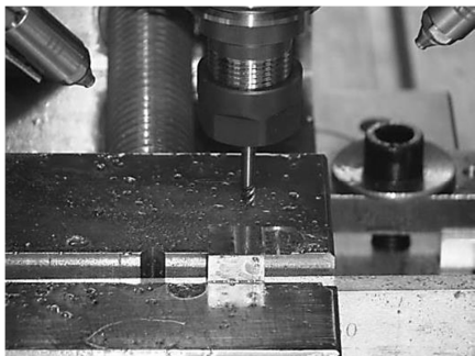
شکل ۱ چیدمان قطعه در آزمایش و موقعیت نازل‌های پاشش روان‌کار
