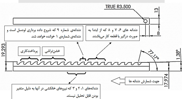
شکل ۴ مشخصات و زوایای سوزن خان‌کش و توضیحات شماره‌ی دندانه‌ها
