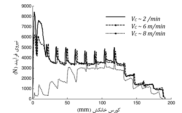
شکل ۹ نمودار تغییرات نیروی وارد شده به ابزار خان‌کشی در سرعت‌های برشی مختلف
