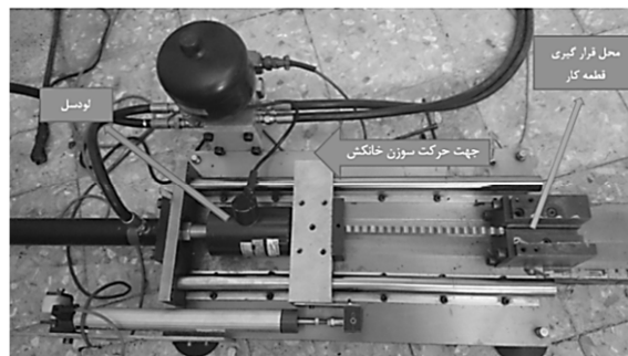
شکل ۷: نحوه‌ی چیدمان اجزای سیستم و جهت حرکت سوزن
