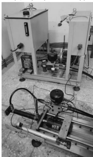
شکل ۶ ستاپ سیستم آزمایش
