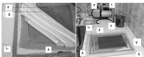
شکل ۳ اجزای فرآیند VARTM؛ ۱- پمپ خلاء ۲- مخزن ایمنی ۳- فشارسنج ۴- لایه توزیع ۵- لایه داکرون ۶- کیسه خلاء ۷- لوله های انتقال رزین ۸- شیرها و اتصالات ۹- لایه جداکننده ۱۰- چسب آب بندی
