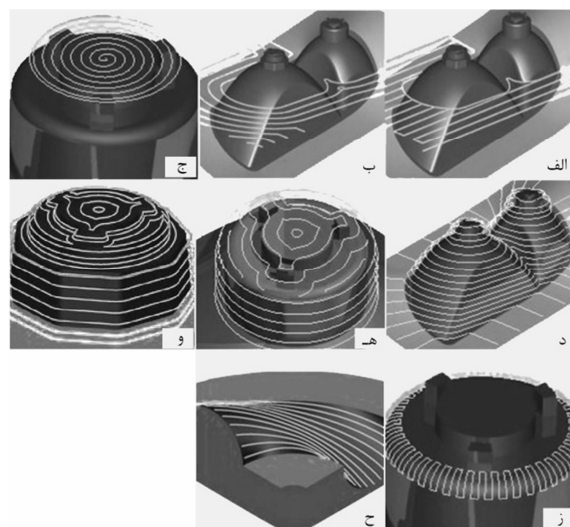
شکل ۱ (الف) رستر (ب) آفست سه‌بعدی (ج) مارپیچ (د) پله‌ای (ه) پله‌ای بهینه‌شده و (پله‌ای تفکیک‌شده (ز) شعاعی (ح) پرداخت سطح
