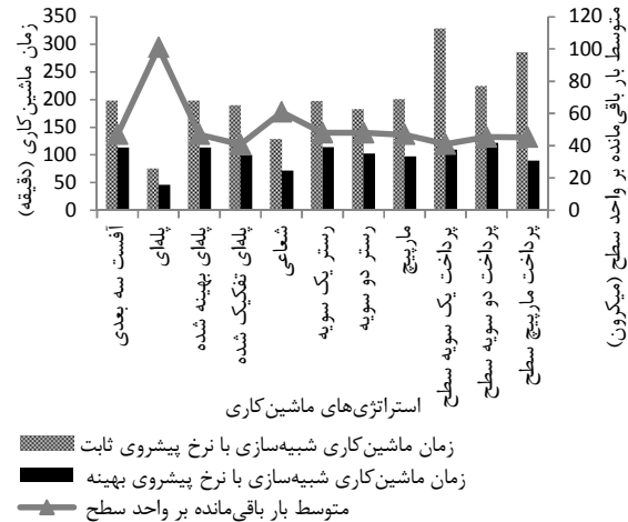
شکل ۸ زمان ماشین کاری و متوسط بار باقی مانده بر واحد سطح حاصل از استراتژی های مختلف برای مدل سطح دارای فرم آزاد
