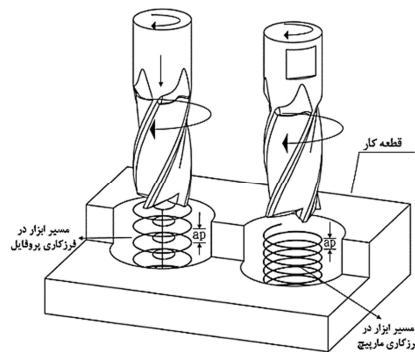
شکل ۱ شماتیک فرزکاری مارپیچ و پروفایل
