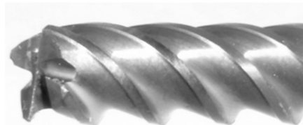
شکل ۷ سایش لبه کناری ابزار استفاده‌شده در فرزکاری پروفایل
