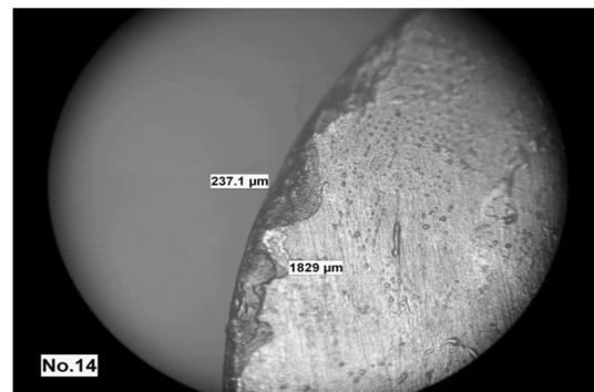
شکل ۳ نمونه‌ای از اندازه‌گذاری سطح براده ابزار سرامیکی
