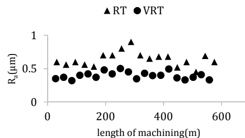
شکل ۳ مقایسه زبری سطح براساس طول ماشین کاری در دو فرآیند VRT و RT
