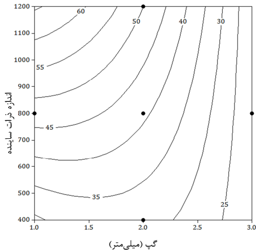
شکل ۱۱ اثر برهم کنش گپ و سایز ذرات ساینده
