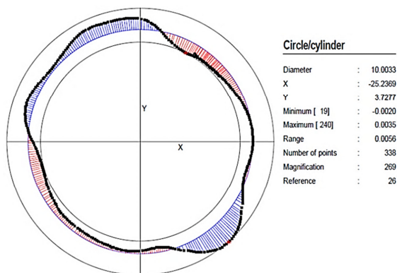
شکل ۲ تلرانس گردی در آزمایش شماره ۸ و ارتفاع ۸ میلی‌متری از سطح سوراخ
