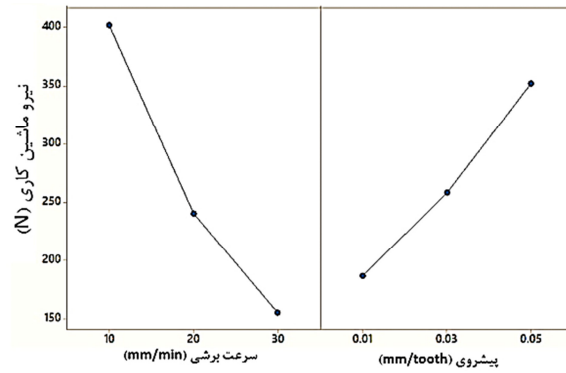
شکل ۱۲ تأثیر پارامترهای برش بر نیروی ماشین کاری در سوراخ کاری معمولی
