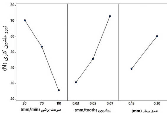
شکل ۵ تأثیر پارامترهای برش بر نیروی ماشین کاری در فرزکاری پروفایل
