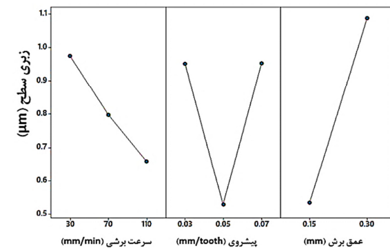
شکل ۱۵ تأثیر پارامترهای برش بر زبری سطح در فرزکاری پروفایل
