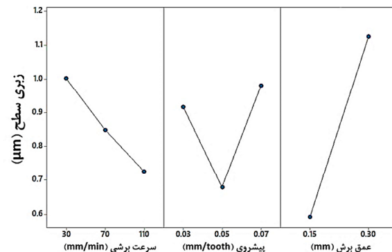
شکل ۱۴ تأثیر پارامترهای برش بر زبری سطح در فرزکاری مارپیچ
