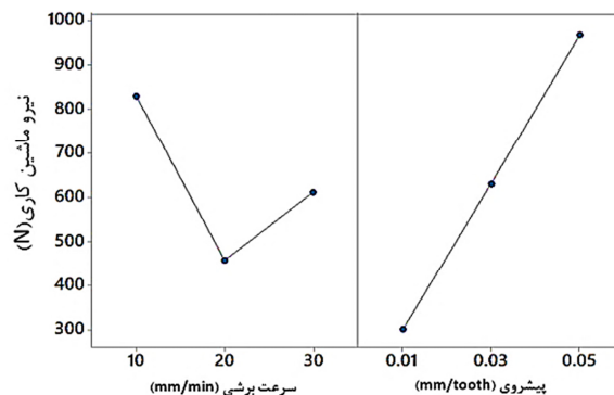
شکل ۱۳ تأثیر پارامترهای برش بر نیروی ماشین کاری در سوراخ کاری با پیش مته نتیجه گیری
