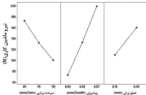
شکل ۴ تأثیر پارامترهای برش بر نیروی ماشین کاری در فرزکاری ماریچ
