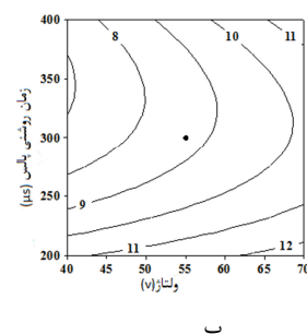
شکل ۹ نمودار دو و سه بعدی ولتاژ و زمان روشنی پالس
