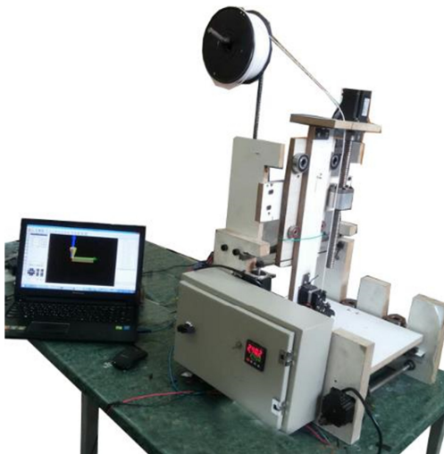
شکل ۵ دستگاه پرینتر سه بعدی ساخته شده
