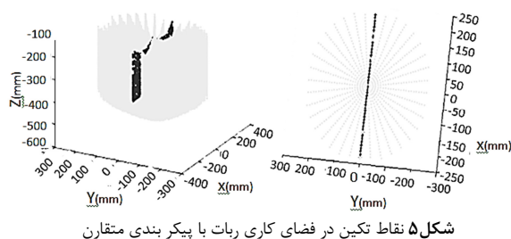
شکل ۵ نقاط تکیه در فضای کاری ربات با پیکر بندی متقارن
