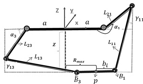
شکل ۴ قرارگیری سکو در بیشترین شعاع
