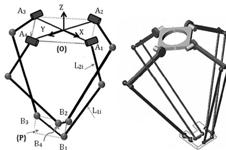
شکل ۱. نمای شماتیک سه بعدی از ربات چهار درجه آزادی
